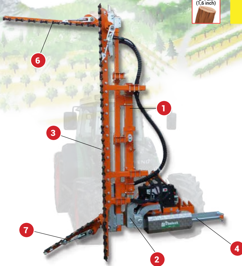
CRF POTATRICE PER FRUTTETO - ORCHARD PRUNING MACHINE- OUTIL DE TAILLE POUR ARBRES FRUITIERS - BAUMSCHNEIDER FÜR DEN SCHNITT UNTER DER KRONE IM OBSTBAU - PODADORA PARA FRUTALES
