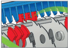
Sistema di taglio con incrocio coltello e controcoltello Cutting blade runs into the counter-blade Schnittsystem Messer-Gegenmesser Sistema de corte con cruce de cuchilla y contra cuchilla Système de coupe avec croisement couteau et contre couteau
