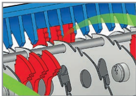
Sistema di taglio con incrocio coltello e controcoltello Cutting blade runs into the counter-blade Schnitssystem Messer-Gegenmesser Sistema de corte con cruce de cuchilla y contra cuchilla Système de coupe avec croisement couteau et contre couteau
